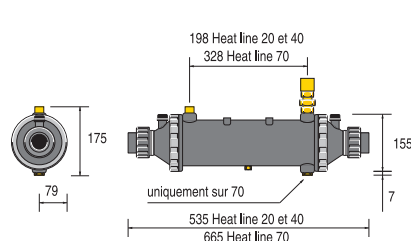
Heat Line neopremiljen
