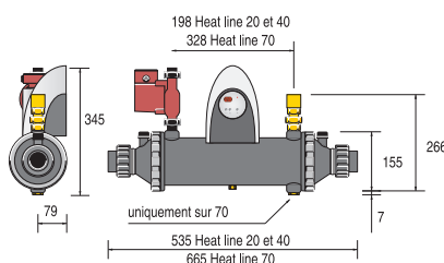
Heat Line Plus sa cirkulacijskom pumpom
