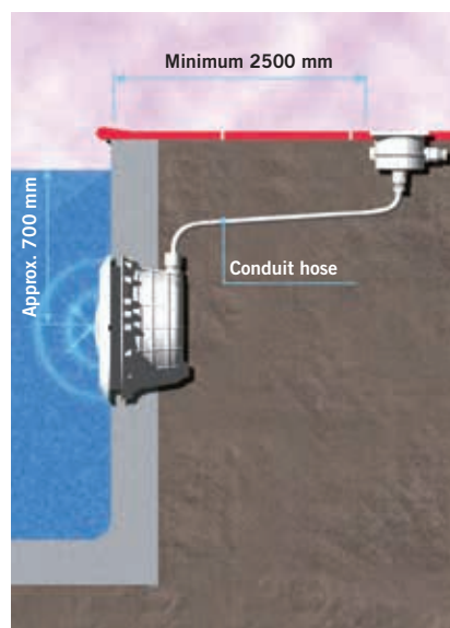
Podvodna ugradnja
