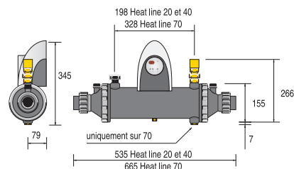
Heat Line Plus bez cirkulacijskom pumpom
