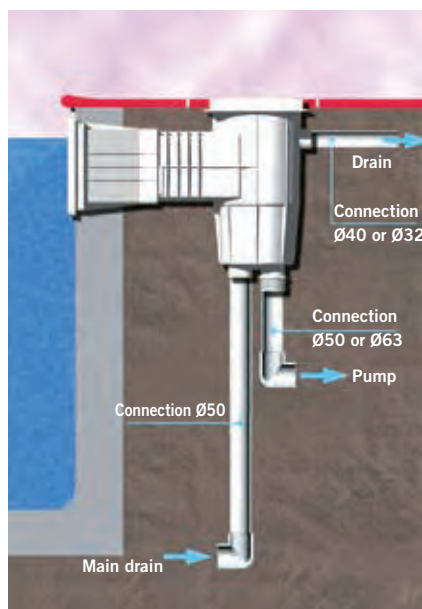
Ugradnja skimera
