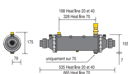
Heat Line neopremiljen
