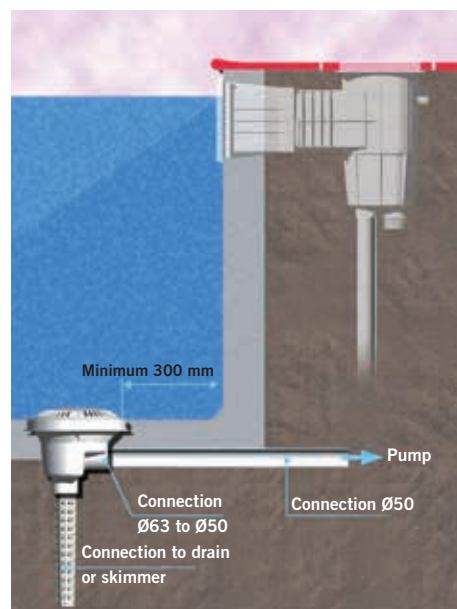
Ugradnja odvoda
