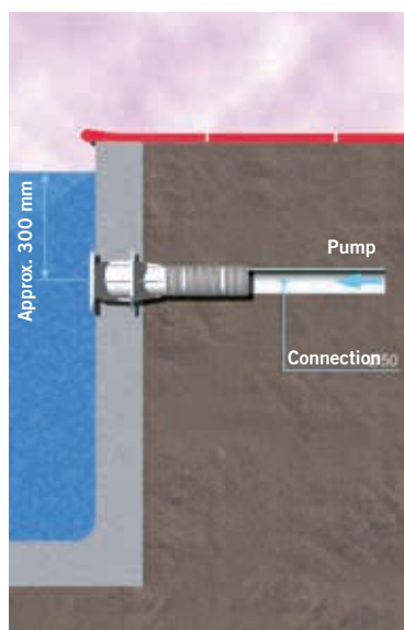
Ugradnja mlaznice
