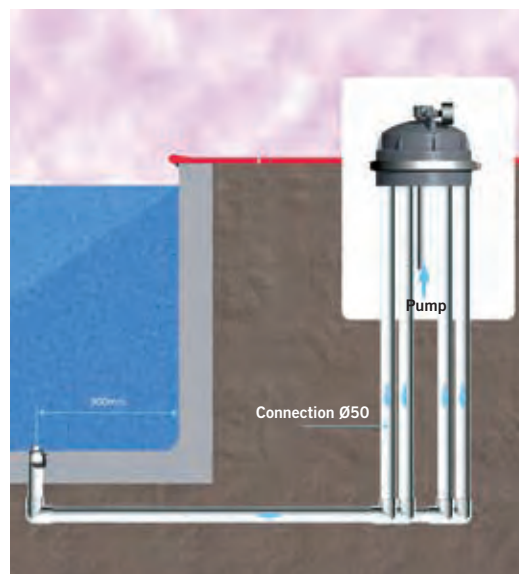
Net'n'Clean ugradnja
