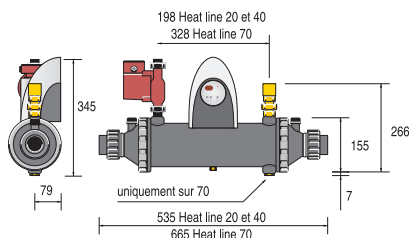
Heat Line Plus sa cirkulacijskom pumpom
